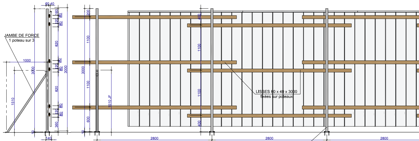
COUPE
