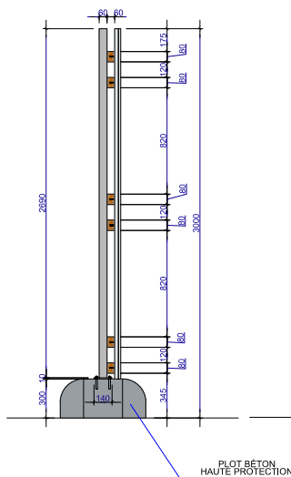
COUPE
