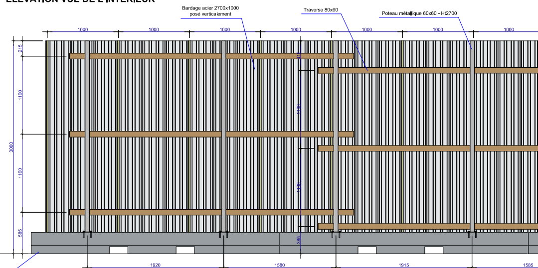
ELEVATION VUE DE L'INTERIEUR
