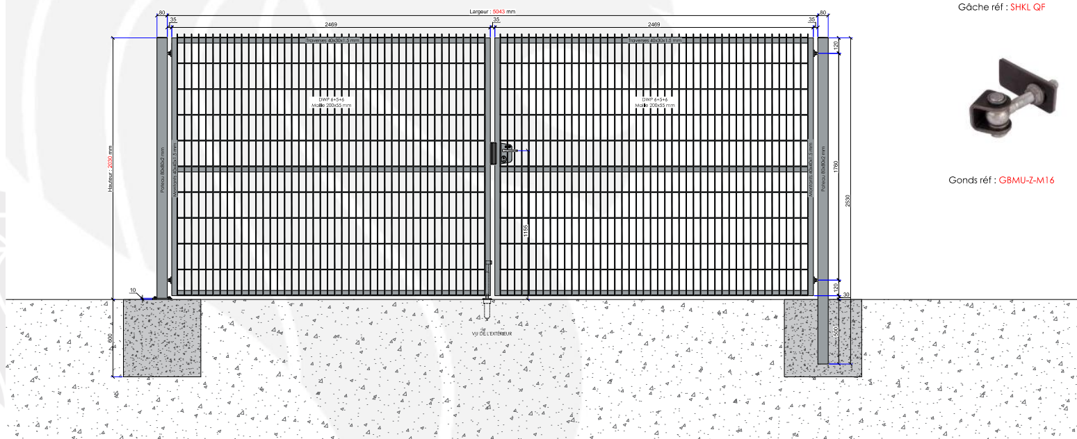
Gâche réf : SHKL QF
